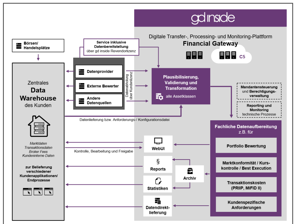
Prozessdarstellung Financial Gateway Transfer-, Processing- und Monitoring-Plattform
