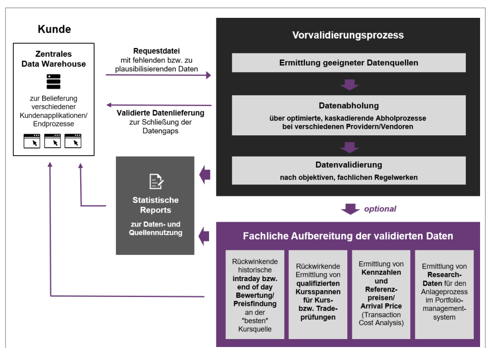
Prozessdarstellung Validation on Demand Service (VDS)
